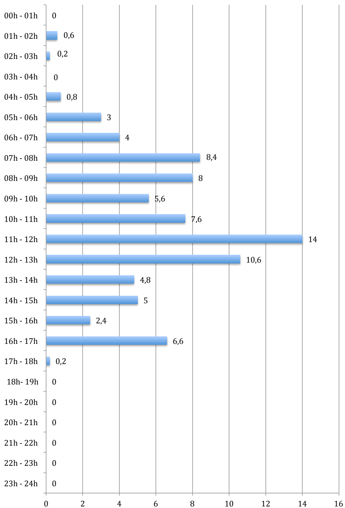
Cantidades de lluvia registradas por horas en BENIGÀNIM el día 19/11/18 (en l/m^2 )
